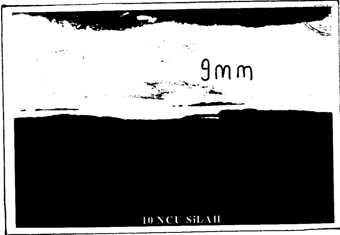
FOTOĞRAF 122-123: GÖVDESİNİN SOL YAN TARAFINDA OLMASI GEREKEN İBARE VE SERİ NUMARALARI KAZINMAK SURETİYLE SİLİNEN 10 NUMARALI MAKİNELİ TABANCANIN LABORATUVARIMIZDA YAPILAN KİMYASAL AŞINDIRMA METODU SAFHALARI İLE TESPİT EDİLEBİLEN İBARE VE NUMARALAR.
