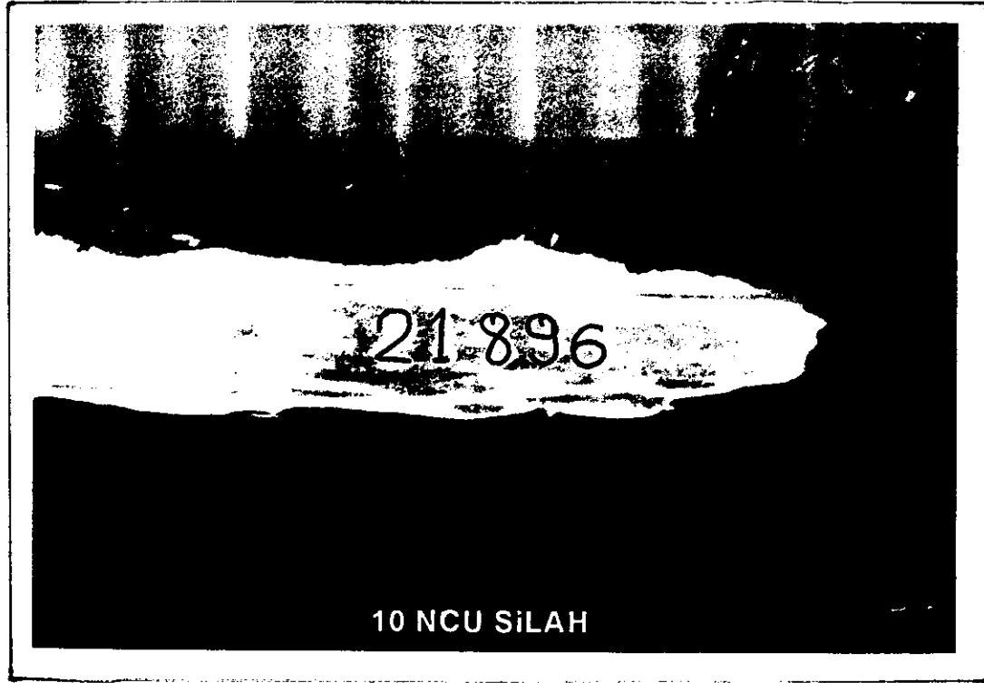
FOTOĞRAF 124-125: GÖVDESİNİN SOL YAN TARAFINDA OLMASI GEREKEN İBARE VE SERİ NUMARALARI KAZINMAK SURETİYLE SİLİNEN 10 NUMARALI MAKİNELİ TABANCANIN LABORATUVARIMIZDA YAPILAN KİMYASAL AŞINDIRMA METODU SAFHALARI İLE TESPİT EDİLEBİLEN İBARE VE NUMARALAR.
