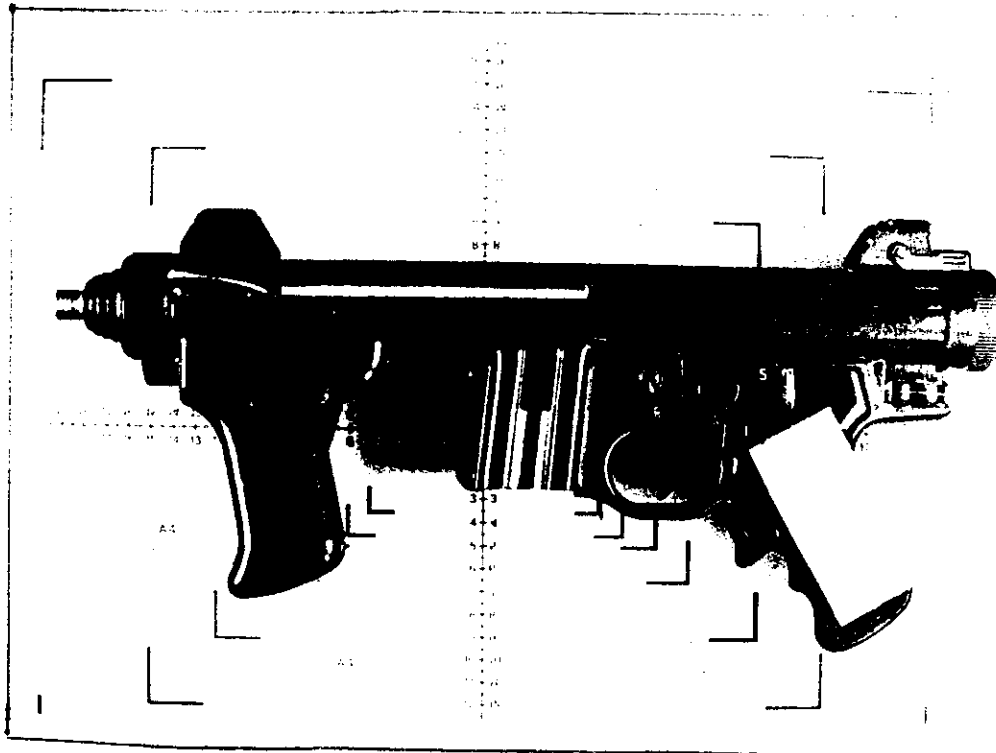
FOTOĞRAF 1-2 :ÜZERİNDEKİ NUMARA VE İBARELERİ KAZINMAK SURETİYLE YOK EDİLMİŞ, 9MM. ÇAPINDA, İTALYA YAPISI, BERETTA MARKA 12 S MODELİ MAKİNELİ TABANCANIN GENEL GÖRÜNÜMÜ (1 NUMARALI SİLAH)
