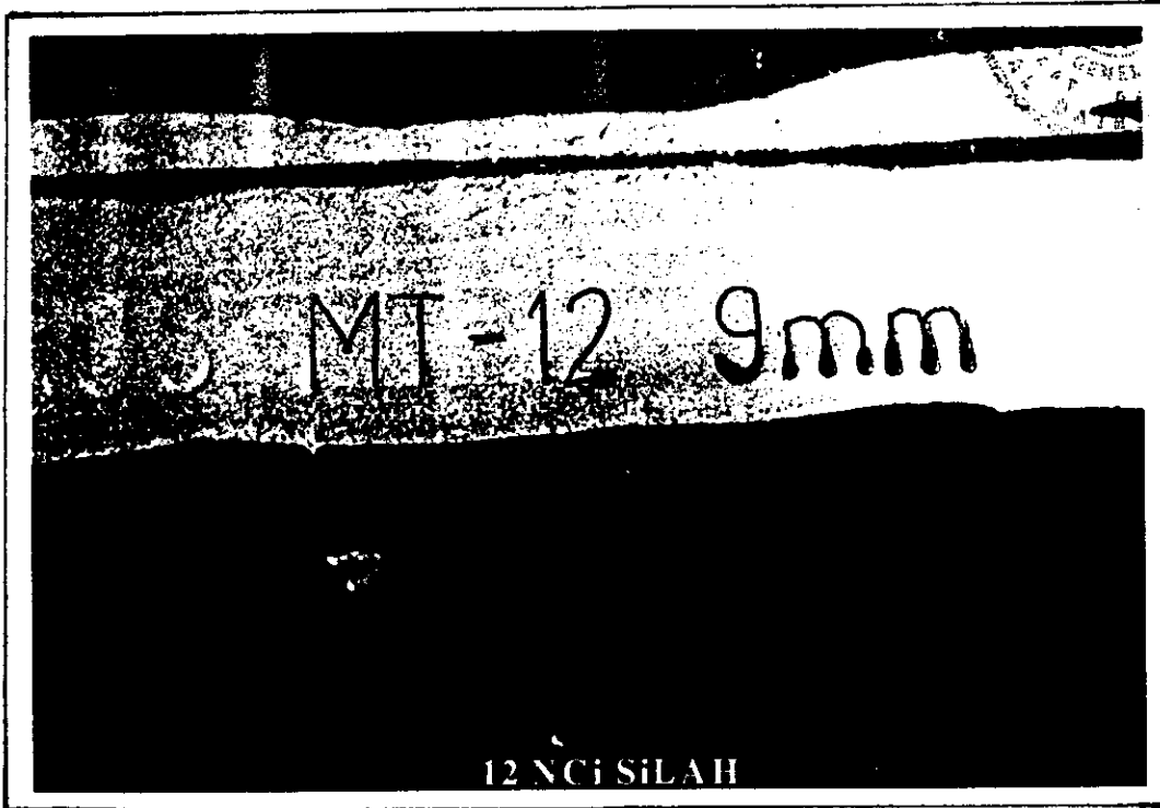
FOTOĞRAF 134-135 : GÖVDESİNİN SOL YAN TARAFINDA OLMASI GEREKEN İBARE VE SERİ NUMARALARI KAZINMAK SURETİYLE SİLİNEN 12 NUMARALI MAKİNELİ TABANCANIN LABORATUVARIMIZDA YAPILAN KİMYASAL AŞINDIRMA METODU SAFHALARI İLE TESPİT EDİLEBİLEN İBARE VE NUMARALAR.
