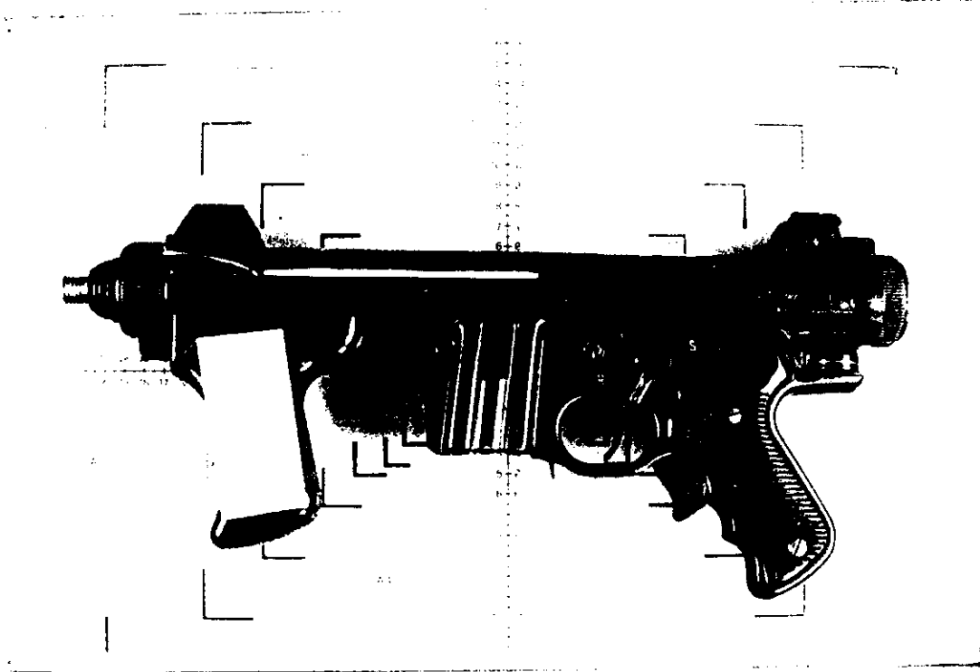
FOTOĞRAF 17-18: ÜZERİNDEKİ NUMARA VE İBARELERİ KAZINMAK SURETİYLE YOK EDİLMİŞ , 9MM. ÇAPINDA, BERETTA MARKA MODEL 12 MAKİNELİ TABANCANIN GENEL GÖRÜNÜMÜ ( 9 NUMARALI SİLAH)
