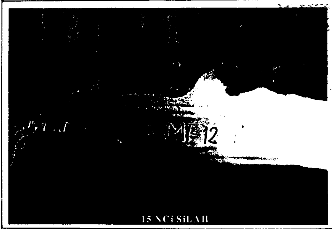
FOTOĞRAF 151-152 : GÖVDESİNİN SOL YAN TARAFINDA OLMASI GEREKEN İBARE VE SERİ NUMARALARI KAZINMAK SURETİYLE SİLİNE 15 NUMARALI MAKİNELİ TABANCANIN LABORATUVARIMIZDA YAPILAN KİMYASAL AŞINDIRMA METODU SAFHALARI İLE TESPİT EDİLEBİLEN İBARE VE NUMARALAR.
