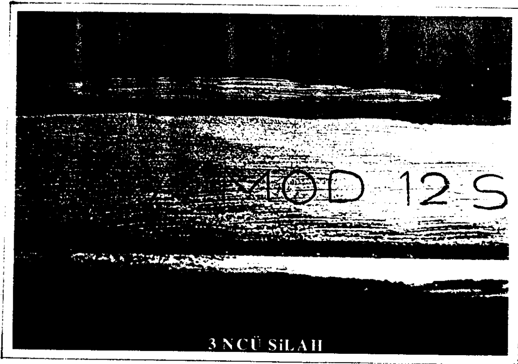
FOTOĞRAF 77-78 : GÖVDESİNİN SOL YAN TARAFINDA OLMASI GEREKEN İBARE VE SERİ NUMARALARI KAZINMAK SURETİYLE SİLİNEN 3 NUMARALI MAKİNELİ TABANCANIN LABORATUVARIMIZDA YAPILAN KİMYASAL AŞINDIRMA METODU SAFHALARI İLE TESPİT EDİLEBİLEN İBARE VE NUMARALAR.
