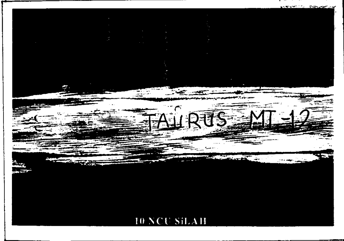
FOTOĞRAF 120-121 : GÖVDESİNİN SOL YAN TARAFINDA OLMASI GEREKEN İBARE VE SERİ NUMARALARI KAZINMAK SURETİYLE SİLİNE 10 NUMARALI MAKİNELİ TABANCANIN LABORATUVARIMIZDA YAPILAN KİMYASAL AŞINDIRMA METODU SAFHALARI İLE TESPİT EDİLEBİLEN İBARE VE NUMARALAR.
