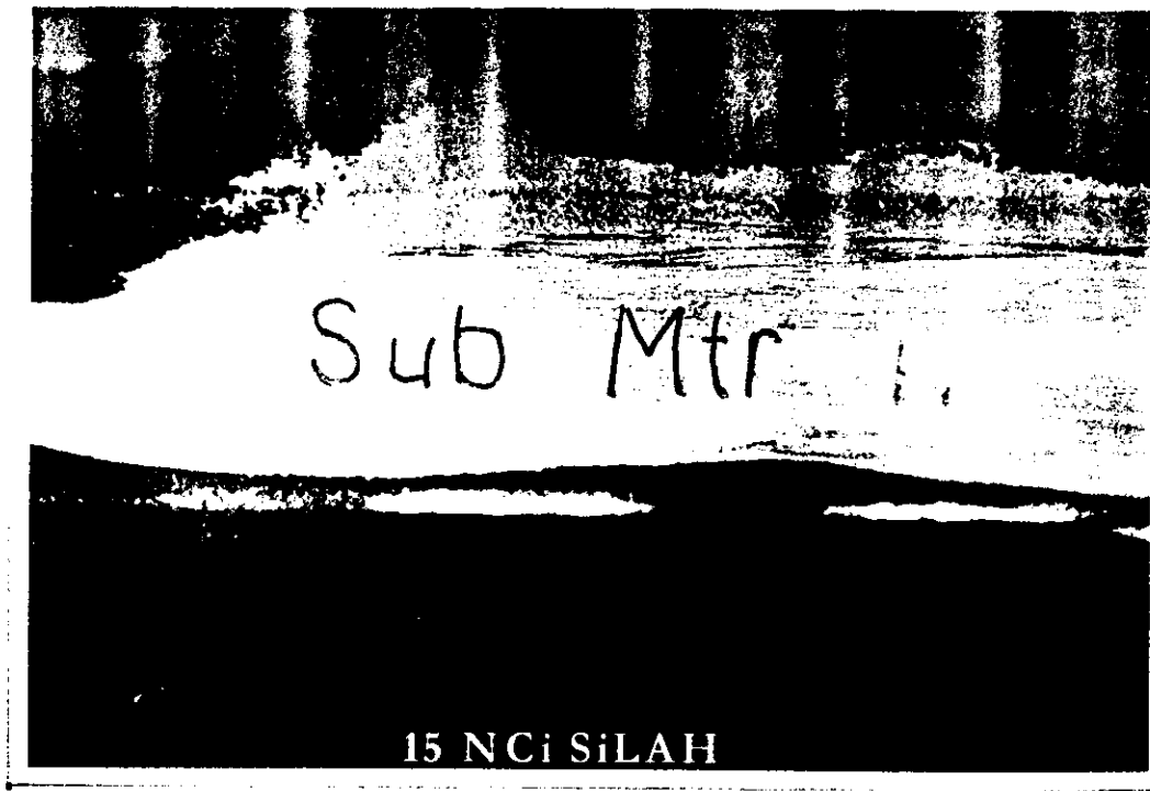
FOTOĞRAF 149-150 : GÖVDESİNİN SOL YAN TARAFINDA OLMASI GEREKEN İBARE VE SERİ NUMARALARI KAZINMAK SURETİYLE SİLİNEN 15 NUMARALI MAKİNELİ TABANCANIN LABORATUVARIMIZDA YAPILAN KİMYASAL AŞINDIRMA METODU SAFHALARI İLE TESPİT EDİLEBİLEN İBARE VE NUMARALAR.
