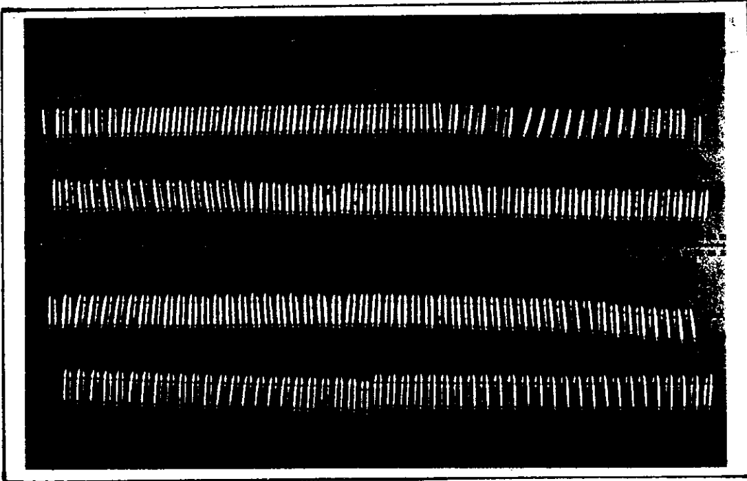
FOTOĞRAF 54 : DÖRTYÜZDOKSANSEKİZ ADET 9X19 95 İBARELİ 9X19 MM. ÇAPINDA FİŞEKTEN İKİYÜZ ADEDİNİN GENEL GÖRÜNÜMÜ
