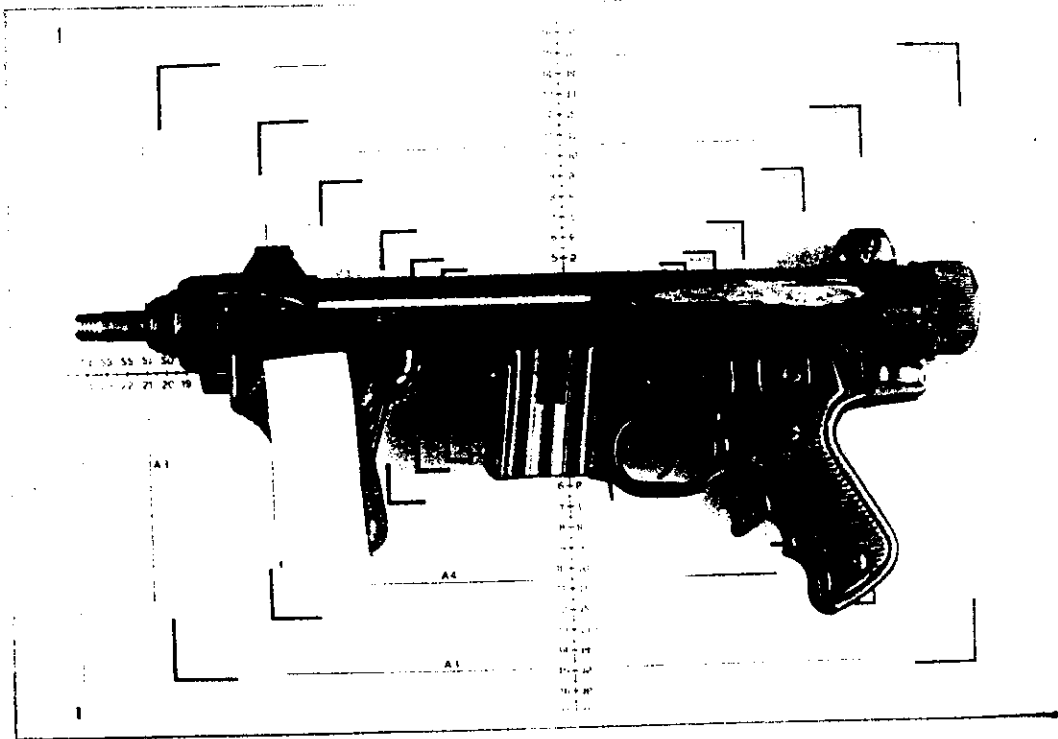
FOTOĞRAF 27-28 :ÜZERİNDEKİ NUMARA VE İBARELERİ KAZINMAK SURETİYLE YOK EDİLMİŞ, 9MM. ÇAPINDA, BREZİLYA YAPISI, BERETTA 12 MODELİ TAURUS MARKA MAKİNELİ TABANCANIN GENEL GÖRÜNÜMÜ ( 14 NUMARALI SİLAH)
