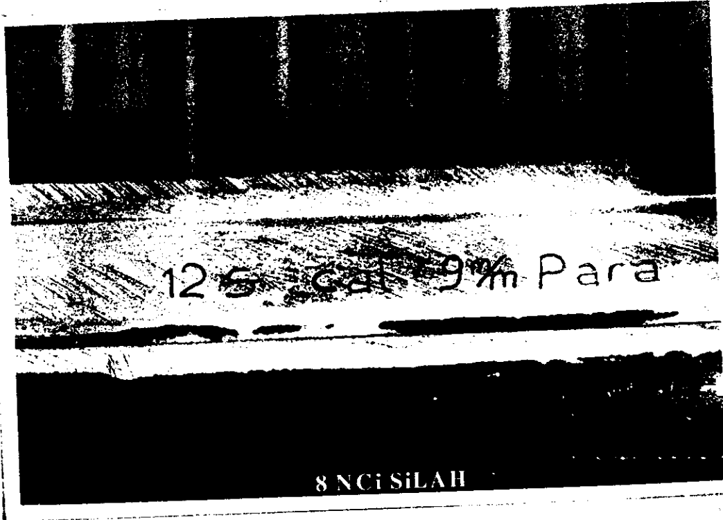
FOTOĞRAF 112-113 : GÖVDESİNİN SOL YAN TARAFINDA OLMASI GEREKEN İBARE VE SERİ NUMARALARI KAZINMAK SURETİYLE SİLİNEN 8 NUMARALI MAKİNELİ TABANCANIN LABORATUVARIMIZDA YAPILAN KİMYASAL AŞINDIRMA METODU SAFHALARI İLE TESPİT EDİLEBİLEN İBARE VE NUMARALAR.
