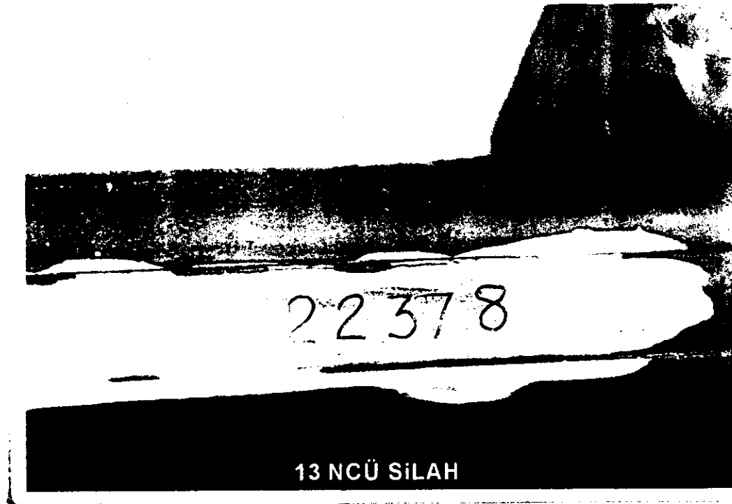
FOTOĞRAF 141-142 : GÖVDESİNİN SOL YAN TARAFINDA OLMASI GEREKEN İBARE VE SERİ NUMARALARI KAZINMAK SURETİYLE SİLİNEN 13 NUMARALI MAKİNELİ TABANCANIN LABORATUVARIMIZDA YAPILAN KİMYASAL AŞINDIRMA METODU SAFHALARI İLE TESPİT EDİLEBİLEN İBARE VE NUMARALAR.
