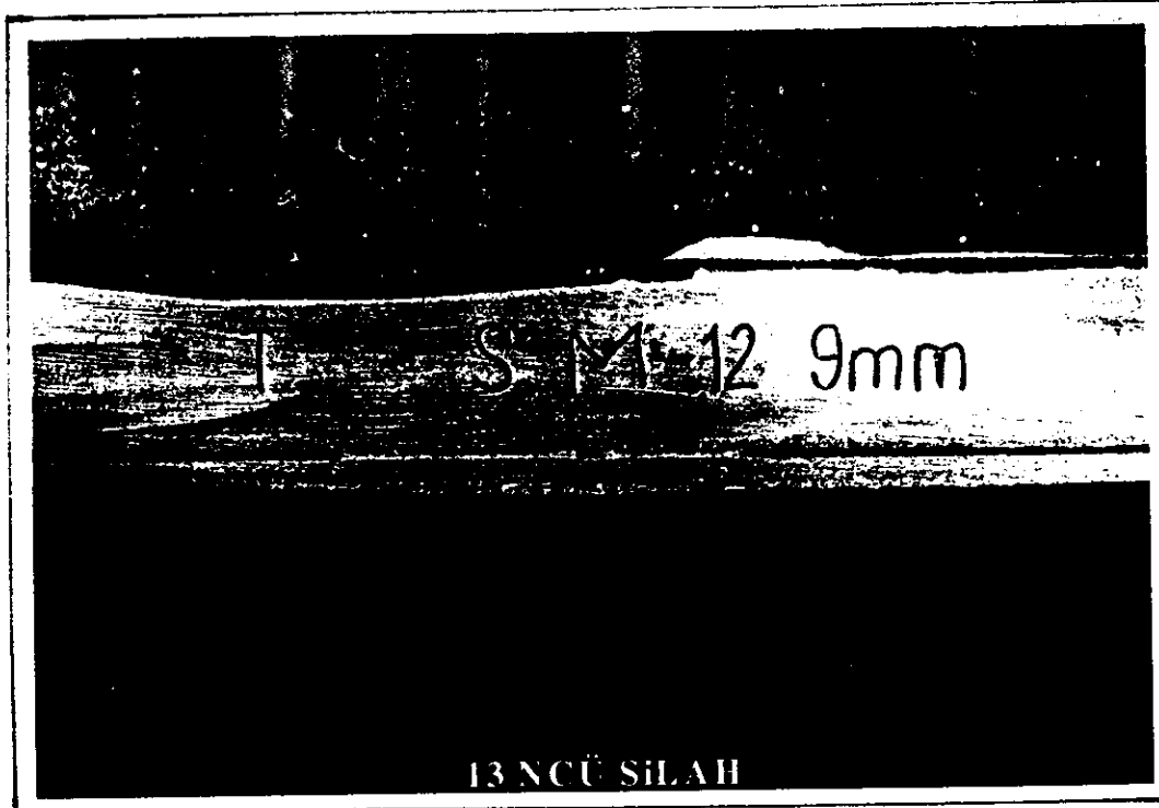
FOTOĞRAF 139-140 : GÖVDESİNİN SOL YAN TARAFINDA OLMASI GEREKEN İBARE VE SERİ NUMARALARI KAZINMAK SURETİYLE SİLİNEN 13 NUMARALI MAKİNELİ TABANCANIN LABORATUVARIMIZDA YAPILAN KİMYASAL AŞINDIRMA METODU SAFHALARI İLE TESPİT EDİLEBİLEN İBARE VE NUMARALAR.
