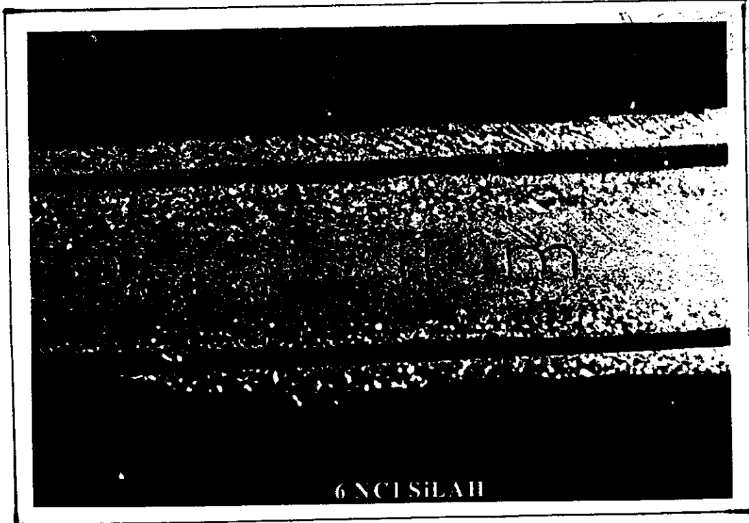
FOTOĞRAF 100-101 : GÖVDESİNİN SOL YAN TARAFINDA OLMASI GEREKEN İBARE VE SERİ NUMARALARI KAZINMAK SURETİYLE SİLİNEN 6 NUMARALI MAKİNELİ TABANCANIN LABORATUVARIMIZDA YAPILAN KİMYASAL AŞINDIRMA METODU SAFHALARI İLE TESPİT EDİLEBİLEN İBARE VE NUMARALAR.
