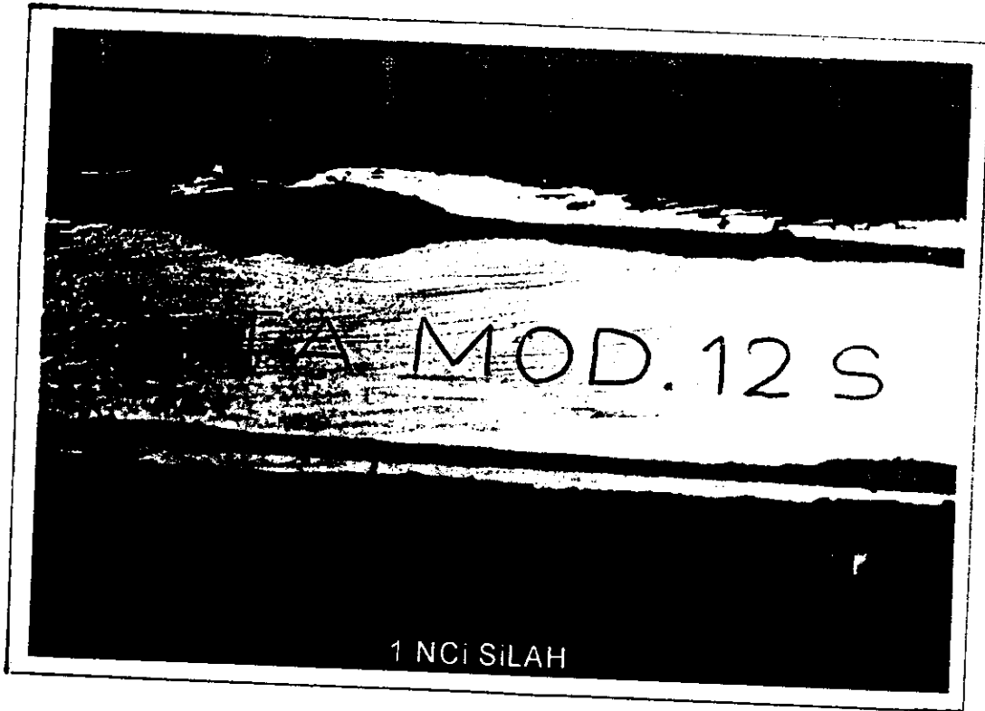
FOTOĞRAF 65-66 : GÖVDESİNİN SOL YAN TARAFINDA OLMASI GEREKEN İBARE VE SERİ NUMARALARI KAZINMAK SURETİYLE SİLİNER 1 NUMARALI MAKİNELİ TABANCANIN LABORATUVARIMIZDA YAPILAN KİMYASAL AŞINDIRMA METODU SAFHALARI İLE TESPİT EDİLEBİLEN İBARE VE NUMARALAR.
