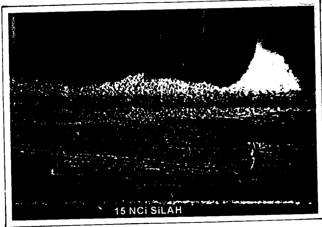
FOTOĞRAF 155-156 : GÖVDESİNİN SOL YAN TARAFINDA OLMASI GEREKEN İBARE VE SERİ NUMARALARI KAZINMAK SURETİYLE SİLİNEN 15 NUMARALI MAKİNELİ TABANCANIN LABORATUVARIMIZDA YAPILAN KİMYASAL AŞINDIRMA METODU SAFHALARI İLE TESPİT EDİLEBİLEN İBARE VE NUMARALAR.
