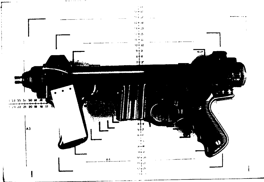
FOTOĞRAF 9-10: ÜZERİNDEKİ NUMARA VE İBARELERİ KAZINMAK SURETİYLE YOK EDİLMİŞ, 9MM. ÇAPINDA, İTALYA YAPISI, BERETTA MARKA 12 S MODELİ MAKİNELİ TABANCANIN GENEL GÖRÜNÜMÜ (5 NUMARALI SİLAH)
