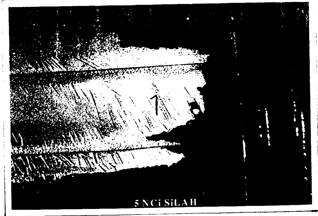
FOTOĞRAF 95-96 : GÖVDESİNİN SOL YAN TARAFINDA OLMASI GEREKEN İBARE VE SERİ NUMARALARI KAZINMAK SURETİYLE SİLİNER 5 NUMARALI MAKİNELİ TABANCA NIN LABORATUVARIMIZDA YAPILAN KİMYASAL AŞINDIRMA METODU SAFHALARI İLE TESPİT EDİLEBİLEN İBARE VE NUMARALAR.
