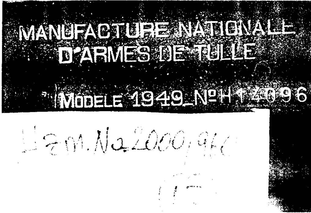
FOTOĞRAF 35 : " H14096 " NUMARALI, 9MM. ÇAPINDA, FRANSA YAPISI, MAT-49 MARKA MAKİNELİ TABANCANIN GENEL GÖRÜNÜMÜ (17 NUMARALI SİLAH)
