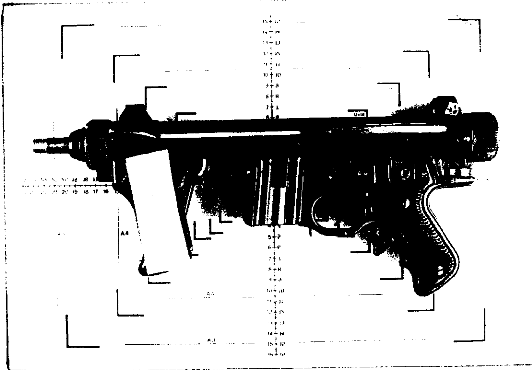
FOTOĞRAF 23-24 : ÜZERİNDEKİ NUMARA VE İBARELERİ KAZINMAK SURETİYLE YOK EDİLMİŞ, 9MM. ÇAPINDA, BREZİLYA YAPISI, BERETTA 12 MODELİ TAURUS MARKA MAKİNELİ TABANCANIN GENEL GÖRÜNÜMÜ ( 12 NUMARALI SİLAH )
