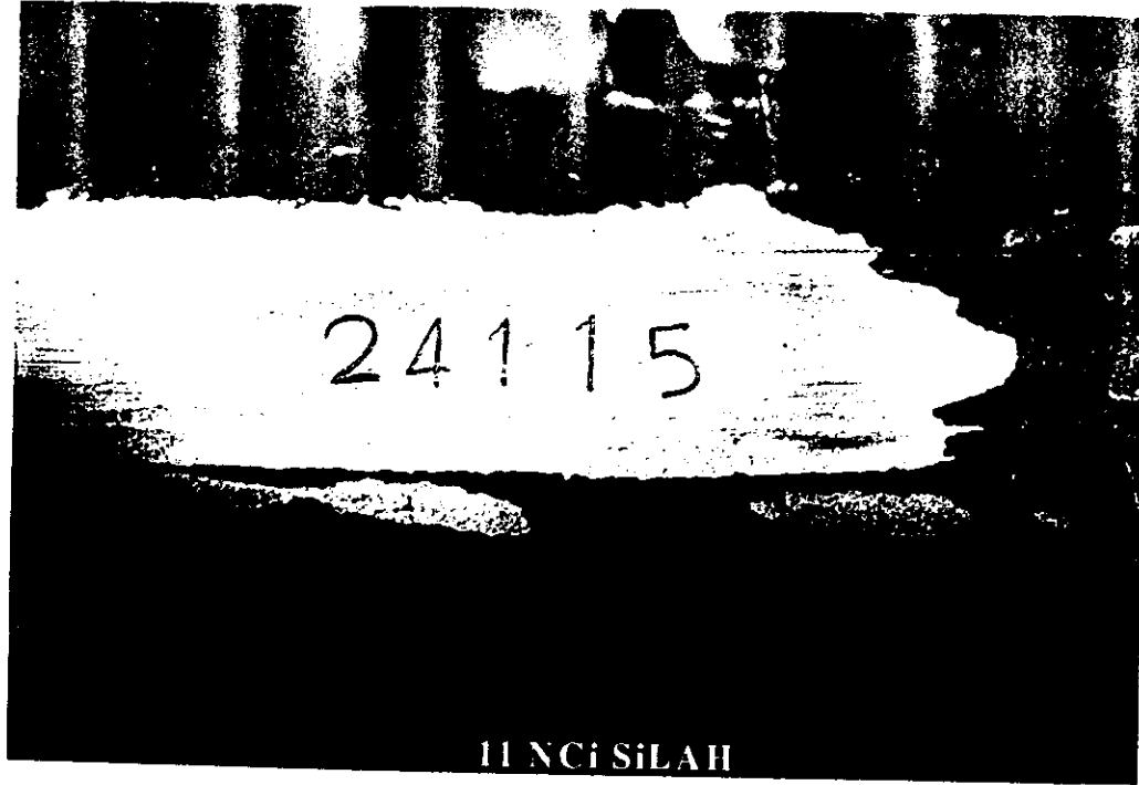
FOTOĞRAF 129-130 : GÖVDESİNİN SOL YAN TARAFINDA OLMASI GEREKEN İBARE VE SERİ NUMARALARI KAZINMAK SURETİYLE SİLİNEN 11 NUMARALI MAKİNELİ TABANCANIN LABORATUVARIMIZDA YAPILAN KİMYASAL AŞINDIRMA METODU SAFHALARI İLE TESPİT EDİLEBİLEN İBARE VE NUMARALAR.
