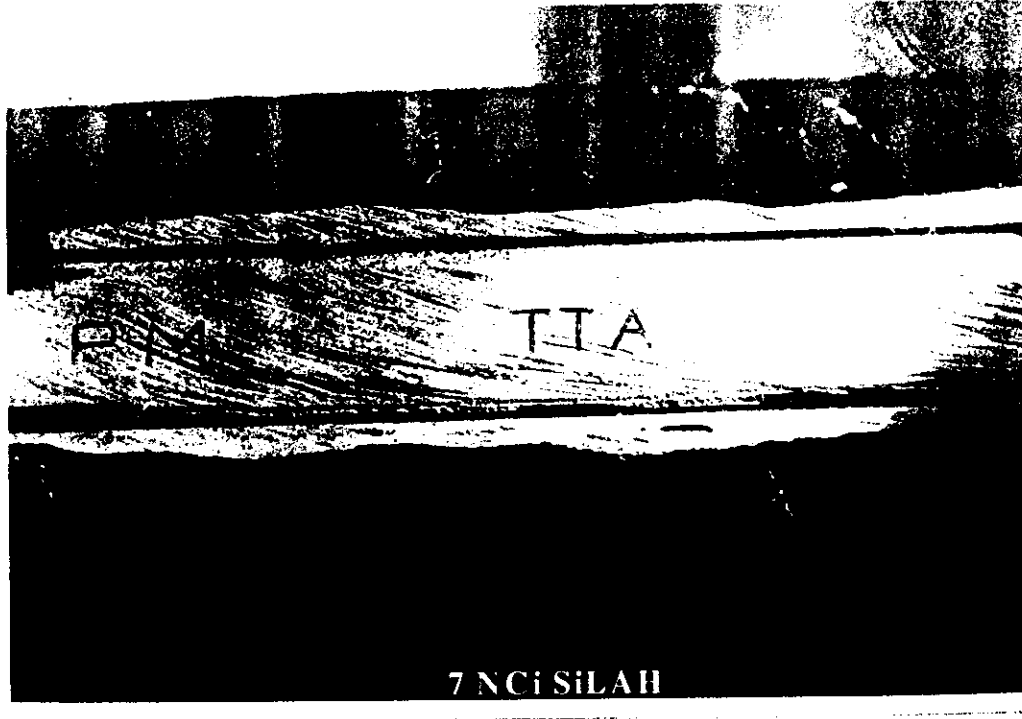
FOTOĞRAF 105-106 : GÖVDESİNİN SOL YAN TARAFINDA OLMASI GEREKEN İBARE VE SERİ NUMARALARI KAZINMAK SURETİYLE SİLİNEN 7 NUMARALI MAKİNELİ TABANCANIN LABORATUVARIMIZDA YAPILAN KİMYASAL AŞINDIRMA METODU SAFHALARI İLE TESPİT EDİLEBİLEN İBARE VE NUMARALAR.
