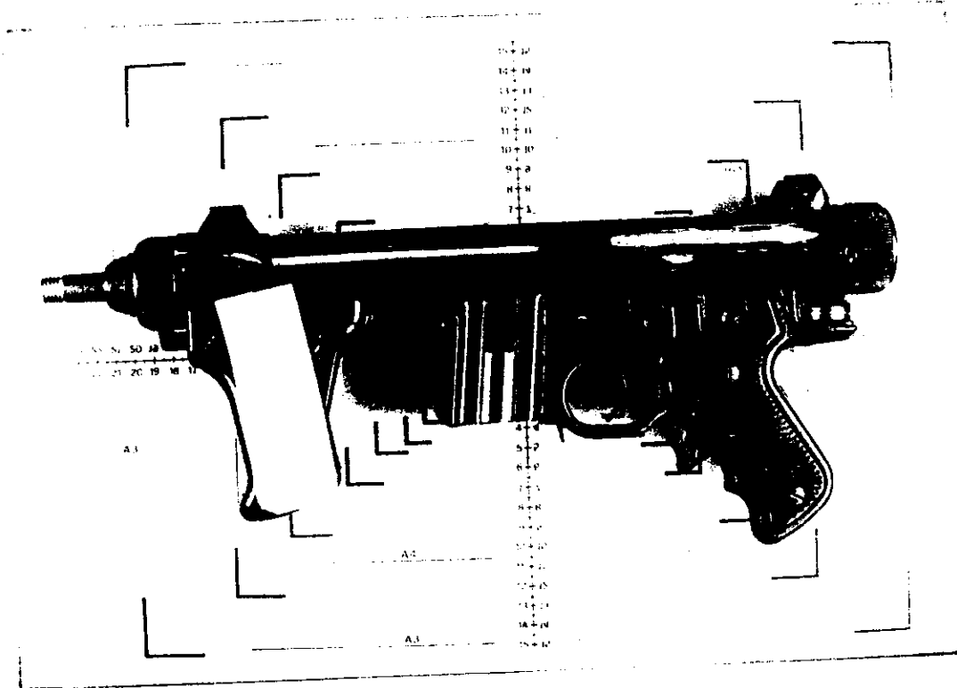
FOTOĞRAF 21-22 :ÜZERİNDEKİ NUMARA VE İBARELERİ KAZINMAK SURETİYLE YOK EDİLMİŞ, 9MM. ÇAPINDA, BREZİLYA YAPISI, BERETTA 12 MODELİ TAURUS MARKA MAKİNELİ TABANCANIN GENEL GÖRÜNÜMÜ ( 11 NUMARALI SİLAH)
